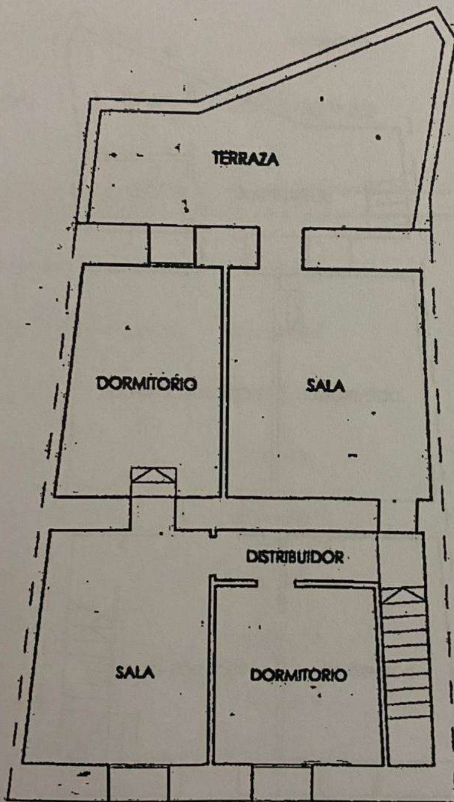
PLANTA PISO
