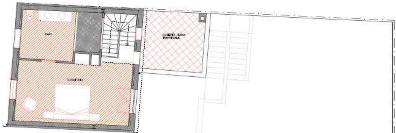
ANEXO PLANTA PISO 2º (DISTRIBUCION)
