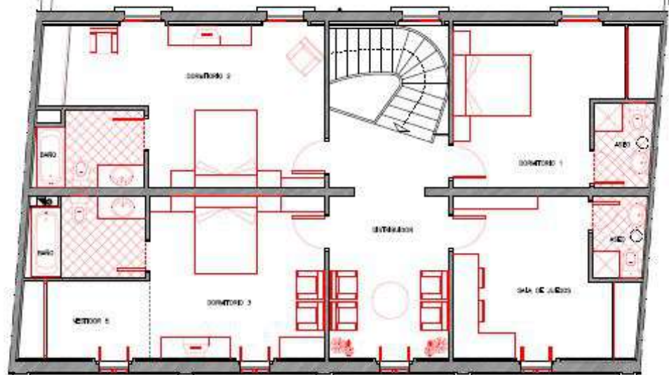
EDIFICIO PRINCIPAL (PLANTA PISO 2º)
